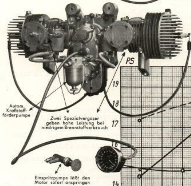
Ansicht von der Vergaserseite
