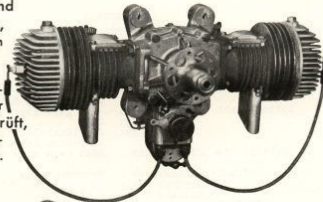
Ansicht von der Vergaserseite
